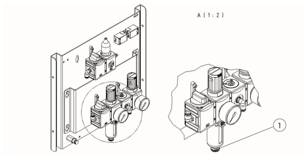
Bild 49: Kondensavtappningsventil tryckluftberedningsenhet
