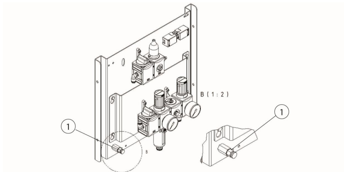
Bild 48: Kondensavtappningsventil tryckluftsbehållare
