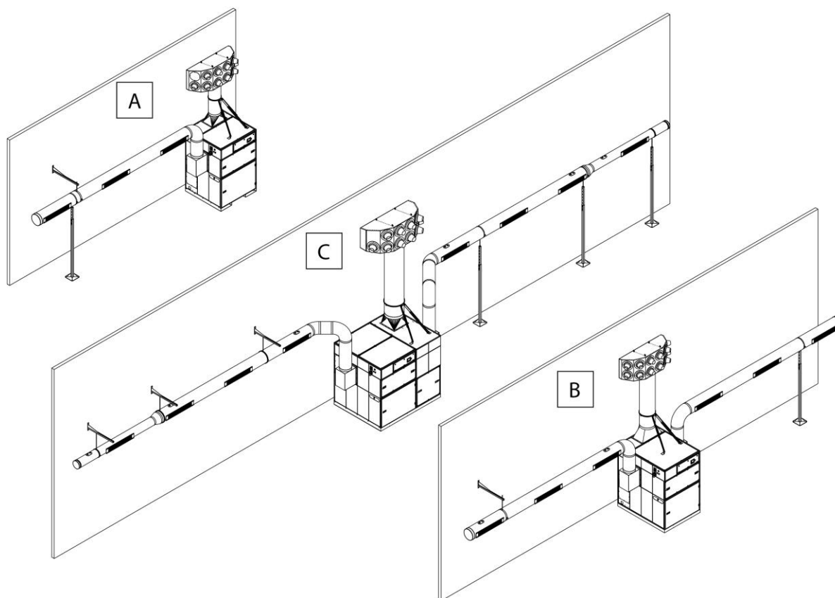
Bild 11: Montering – översikt över produktvarianter
