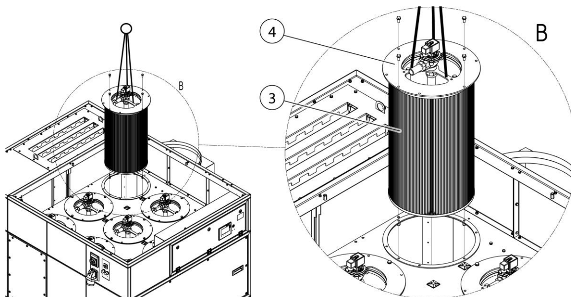
Bild 45: Filterbyte – demontera filterfäste
