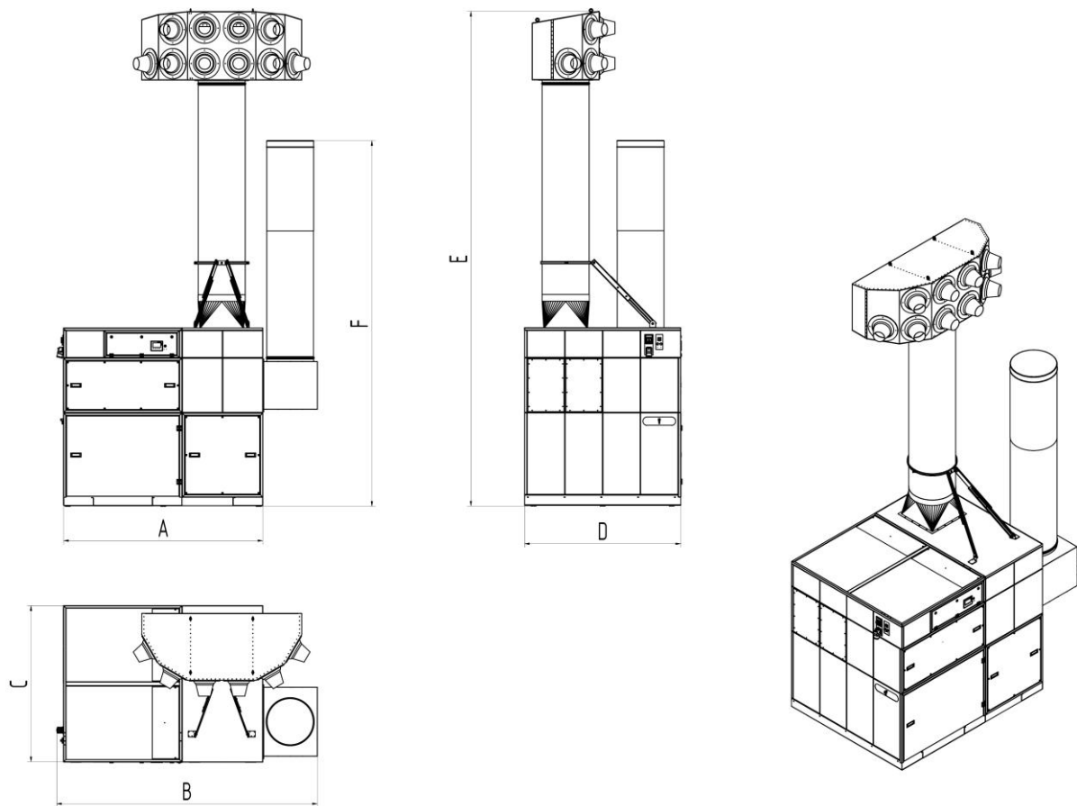
Bild 62: Måttblad - 998800463
