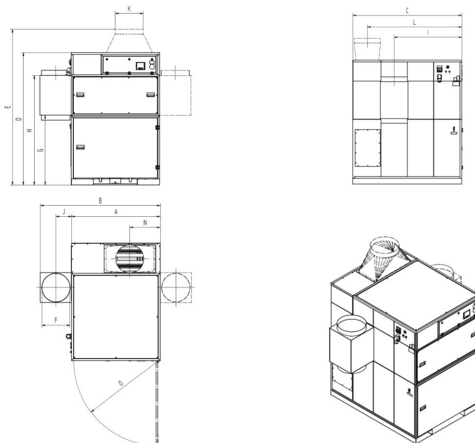
Bild 55: Måttblad 998701371 (998800401, 998800462)
