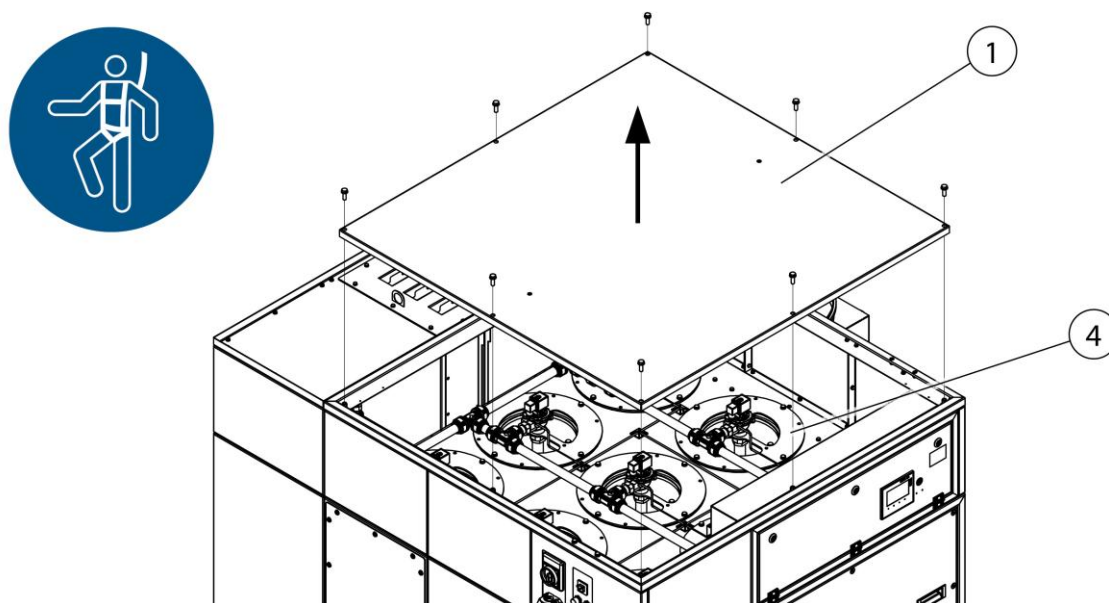
Bild 42: Filterbyte – demontera lockplåt
