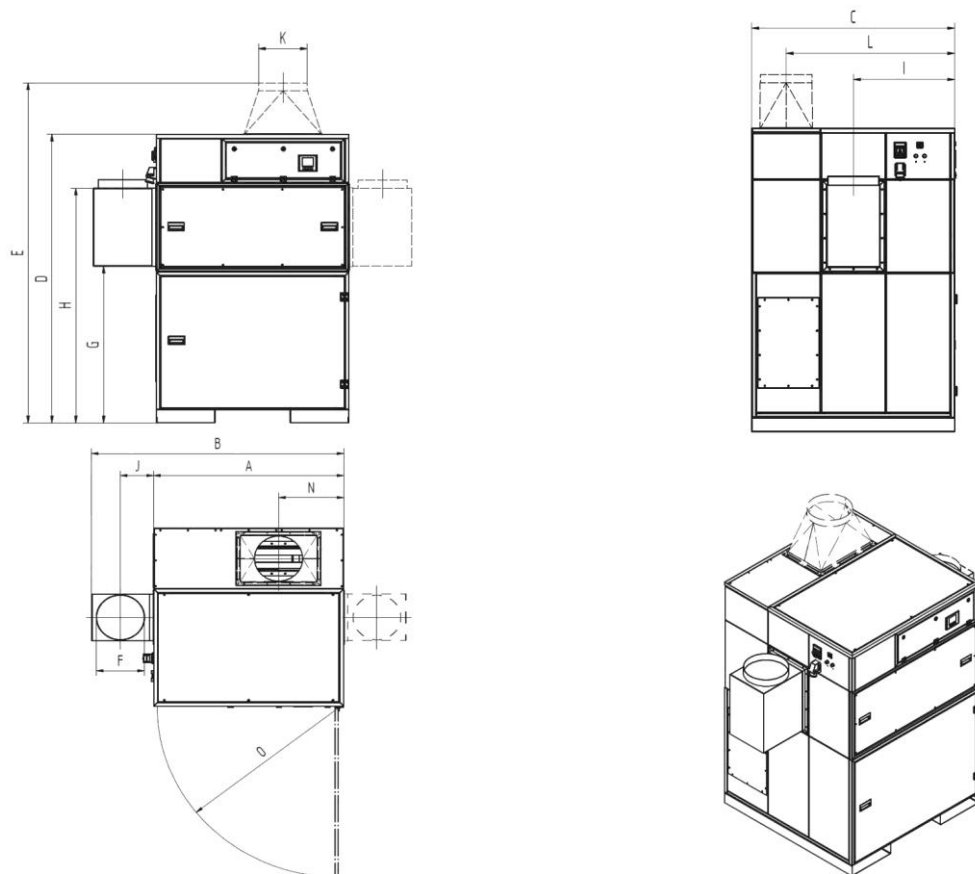
Bild 54: Måttblad 998701372 (998800407, 998800461)
