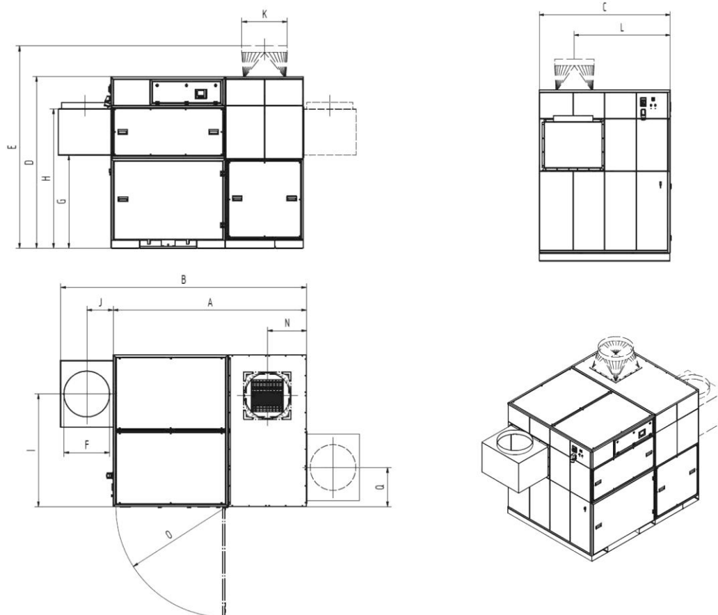
Bild 56: Måttblad 998701370 (998800414, 998800463)
