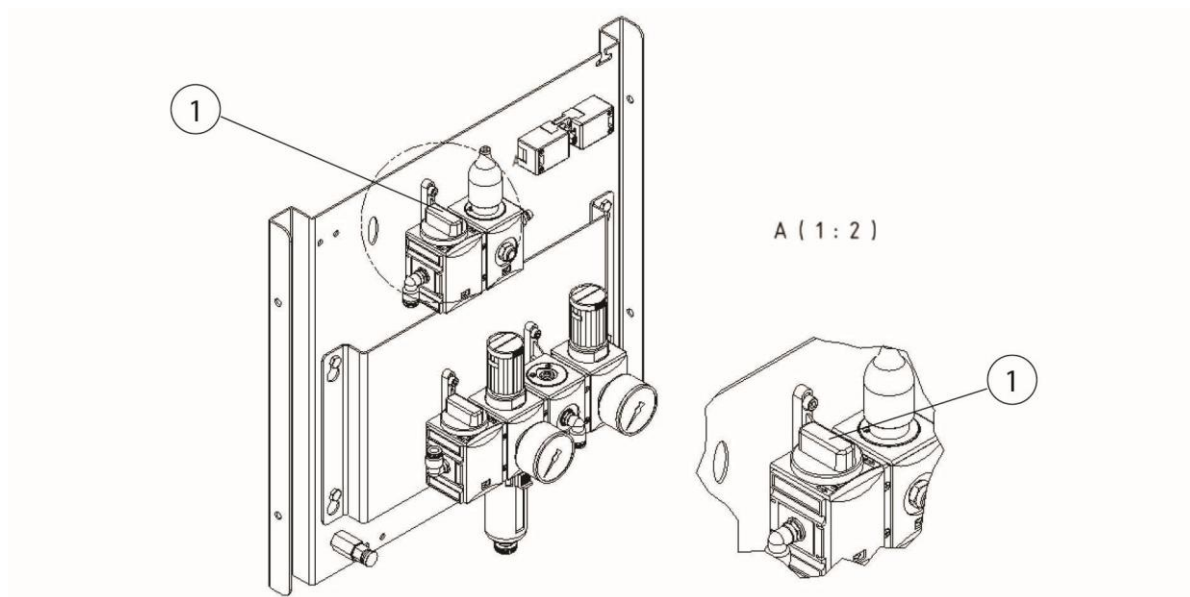
Bild 34: Tryckluftsväventil stoftsamlingsbehållare
