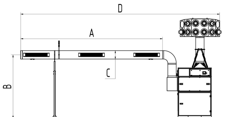
Bild 57: Måttblad – 998800407
