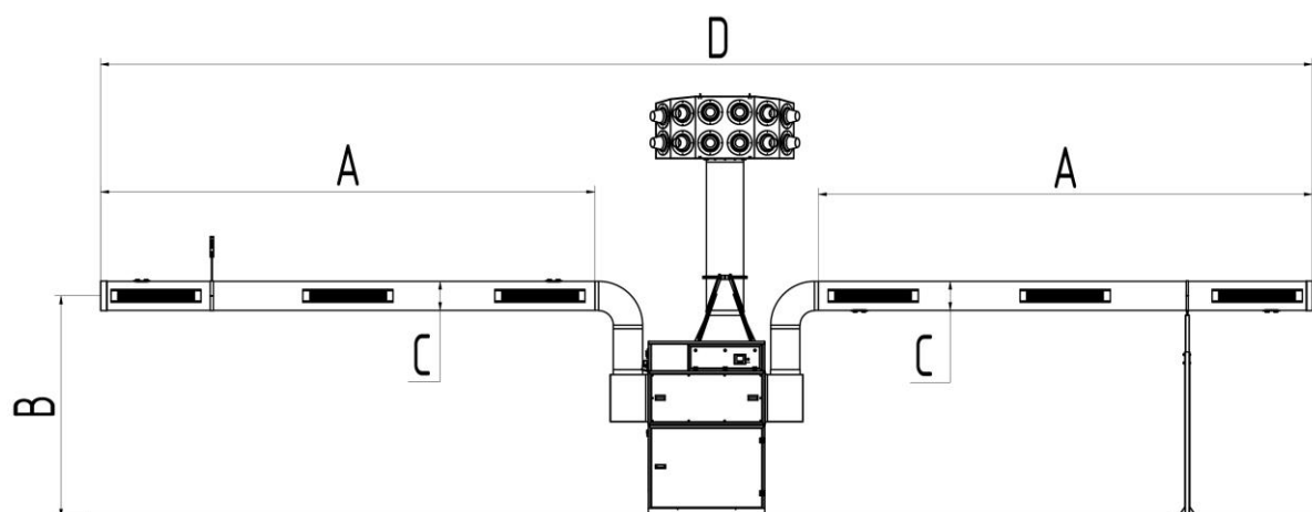
Bild 58: Måttblad – 998800401
