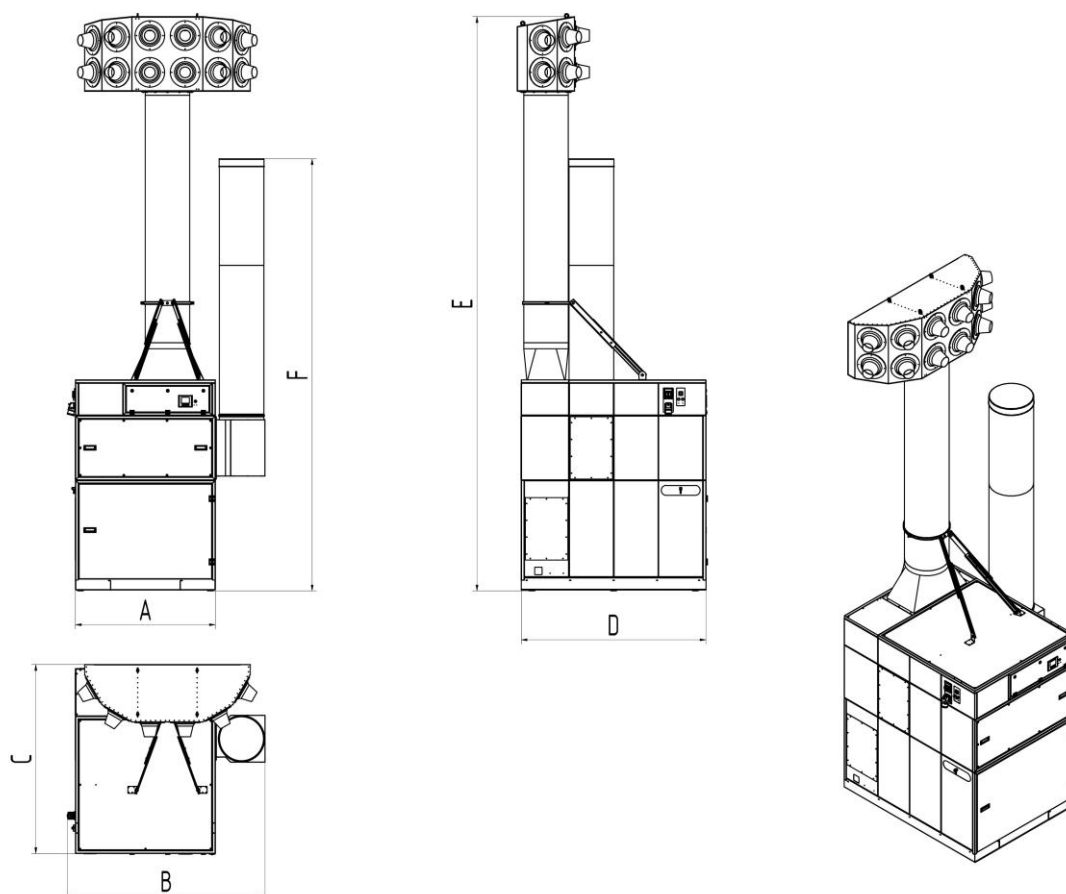
Bild 61: Måttblad – 998800462
