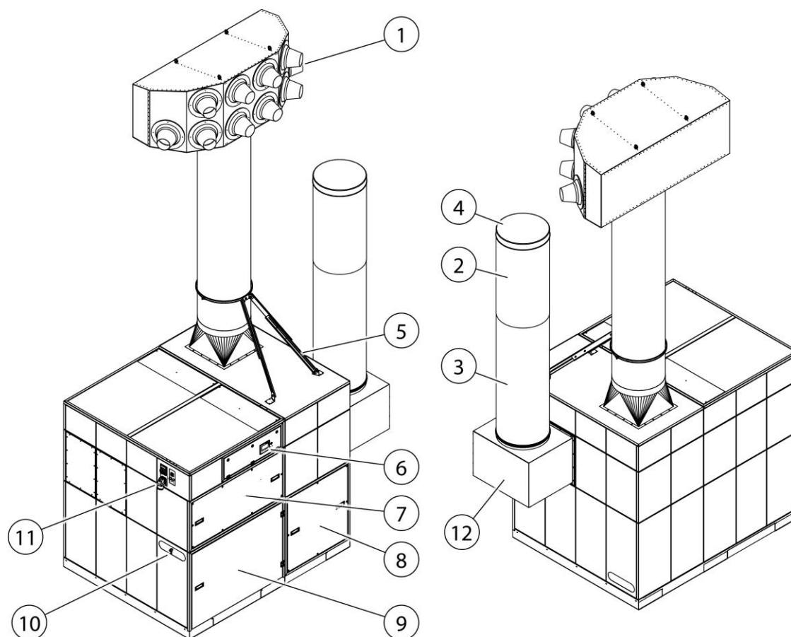
Bild 6: Funktionsbeskrivning – 998800463
